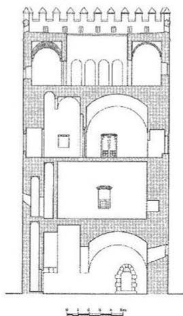
LA ALGABA. TORRE DE LOS GUZMANES. SECCIÓN
